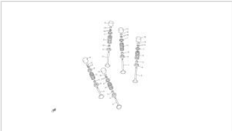
Válvula 450
